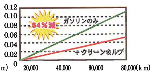
排気ガステスト結果 (窒素酸化物)
